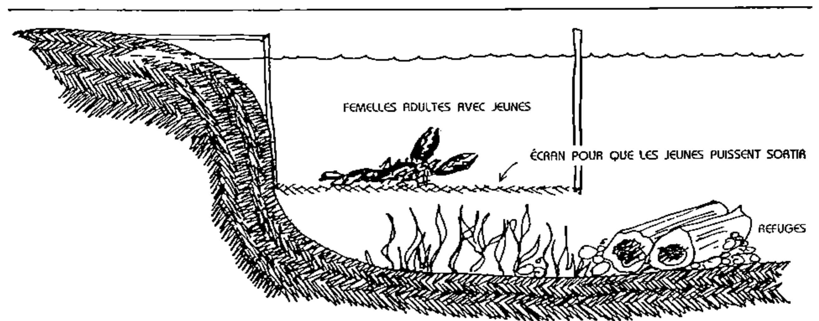
FIG. 7.19 : PANIER A FRAI POUR CRUSTACÉS D'EAU DOUCE PORTANT LEUR OEUFS ET LEURS JEUNES SOUS LA QUEUE (ÉCREVISSÉS, HOMARDS).
