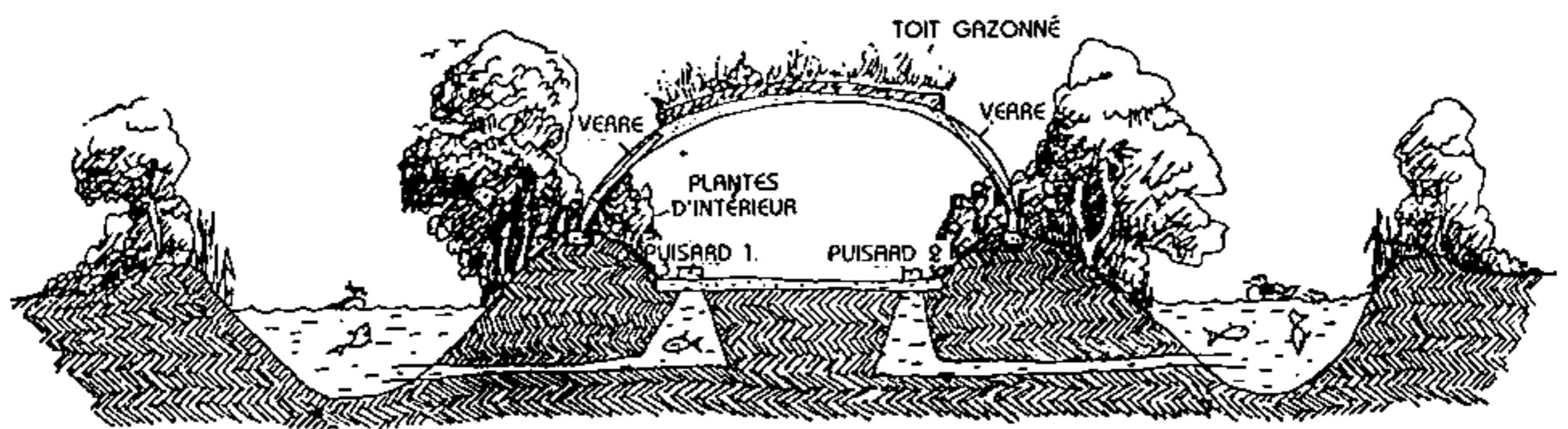
FIG. 6.6 : SECTION D'UNE MAISON EN TERRE — DES DIVISIONS LÉGÈRES PEUVENT ÊTRE ÉTABLIES À L'INTÉRIEUR. LE MUR SUD EST EN VERRRE, LE MUR NORD EST EN TERRE, SANS OUVERTURE.
