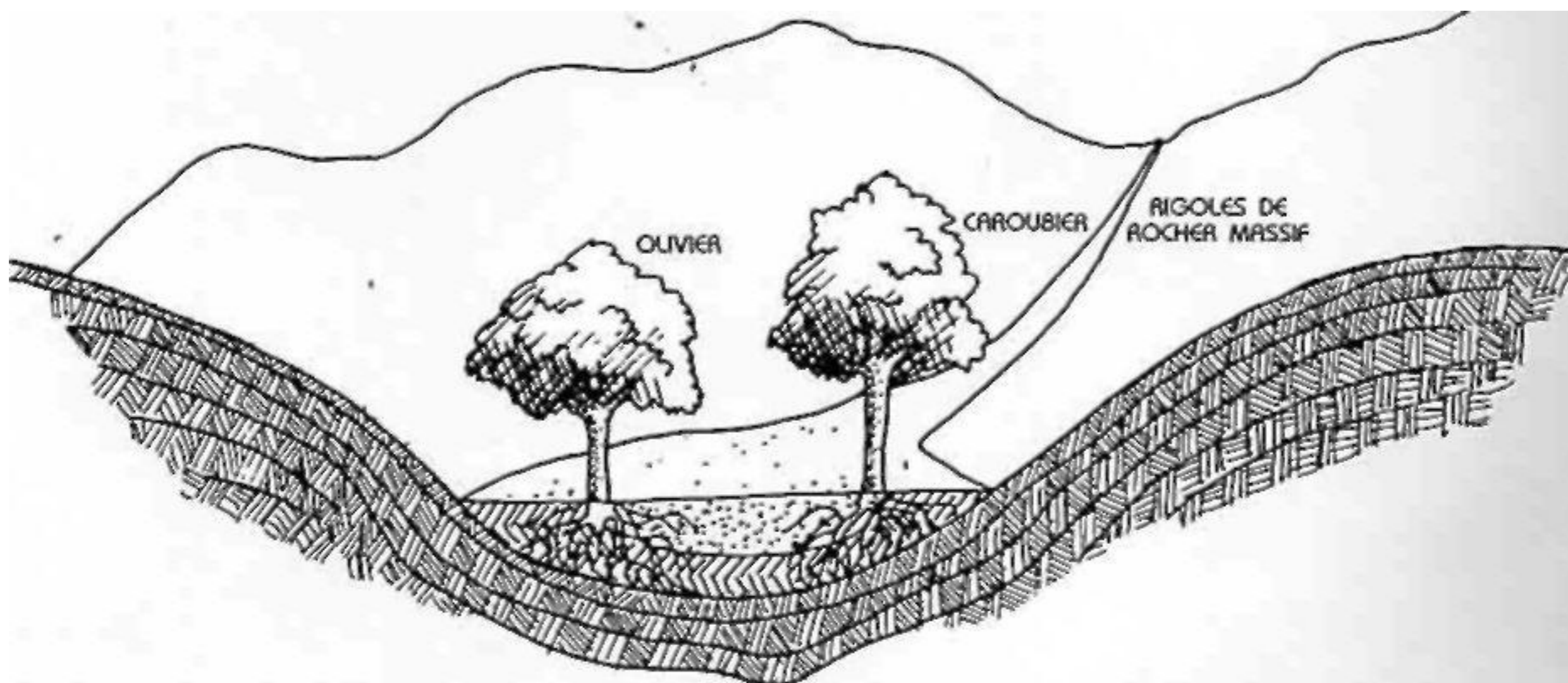
FIG. 5.8 : AU-DESSUS DE KfITJIKfITJIDRRfi : DES RAVINEMENTS DANS LE ROCHER RECUEILLANT DE LA TERRE, DE L'ERU. DES FEUILLES ET DES FIENNES. CES ZONES PEUVENT ETRE SANS T6RMIT6S.
