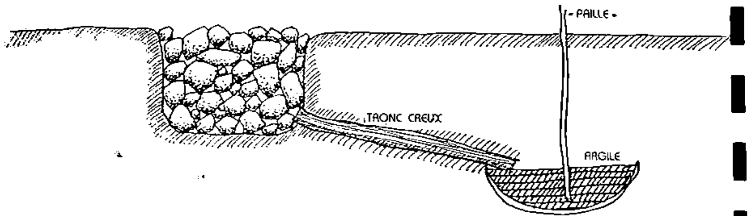
FIG. 5.19 : CONDENSATEUR LOCAL UTILISÉ EN AUSTRALIE OCCIDENTALE (DONNÉES DE PHIL GALL).
