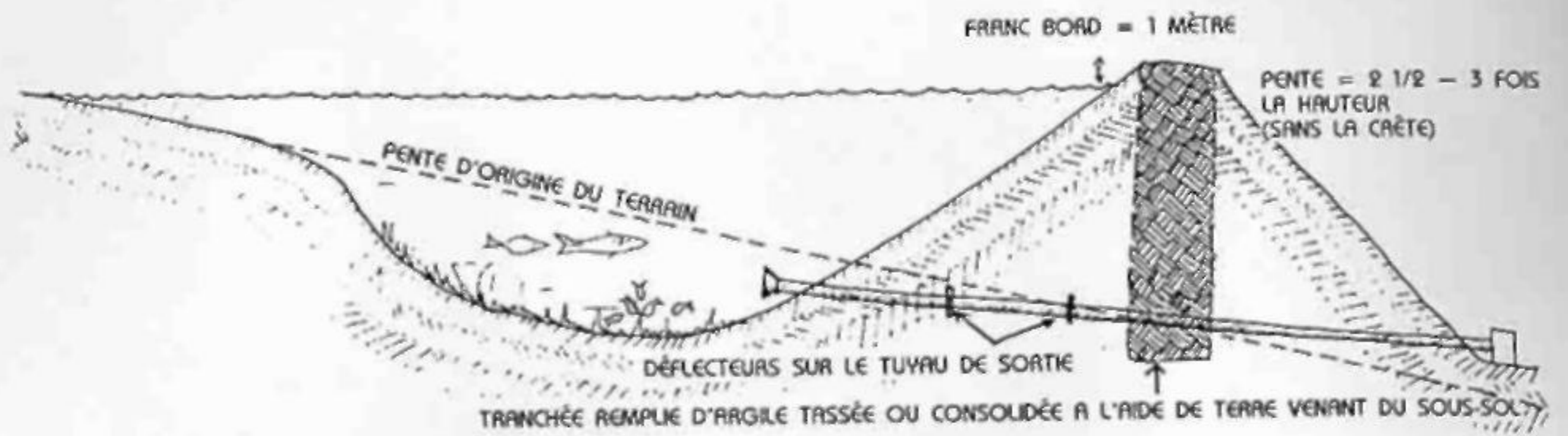
FIG. 7.2 : UN BARRAGE CLASSIQUE (D'APRÈS YEOMANS®). SECTION.
