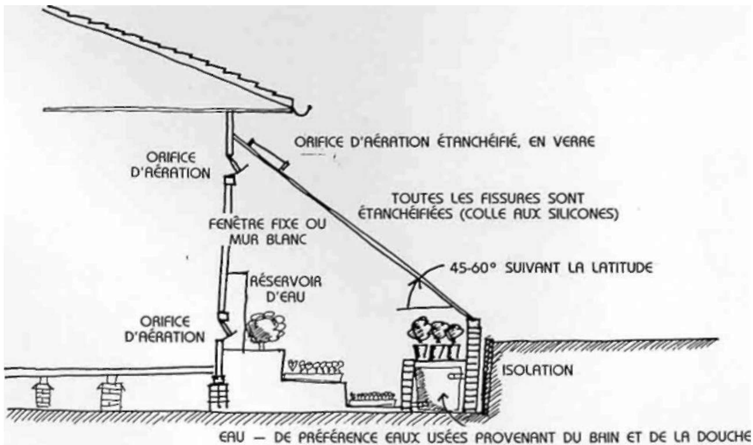
FIG. 6.3 : POINTS PRINCIPAUX DE LA SERRE INTÉGRÉE.
