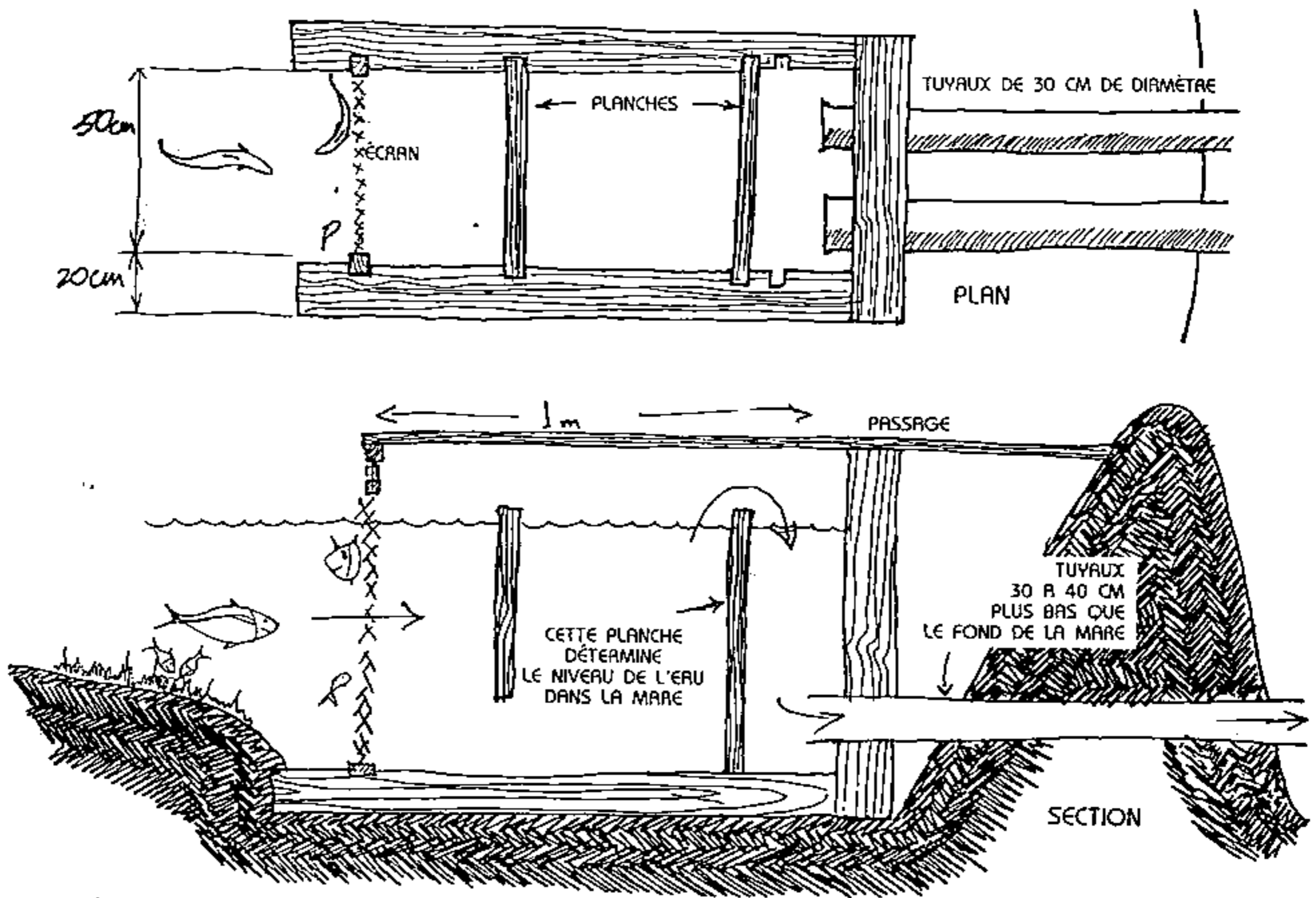
FIG. 7.15 : L'ÉCRAN A POISSONS CLASSIQUE « HERGUTH MONK », AVEC TROP-PLEIN POUR ÉCOULEMENT CONSTANT.
