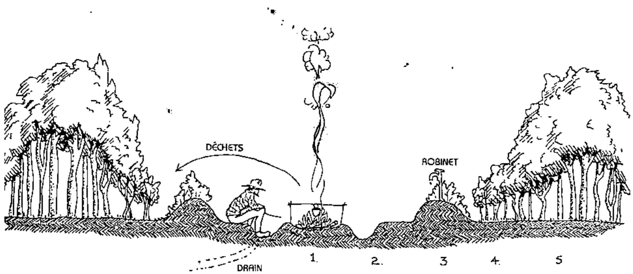
FIG. 6.18 : MANDALA DE FEU (SECTION).
