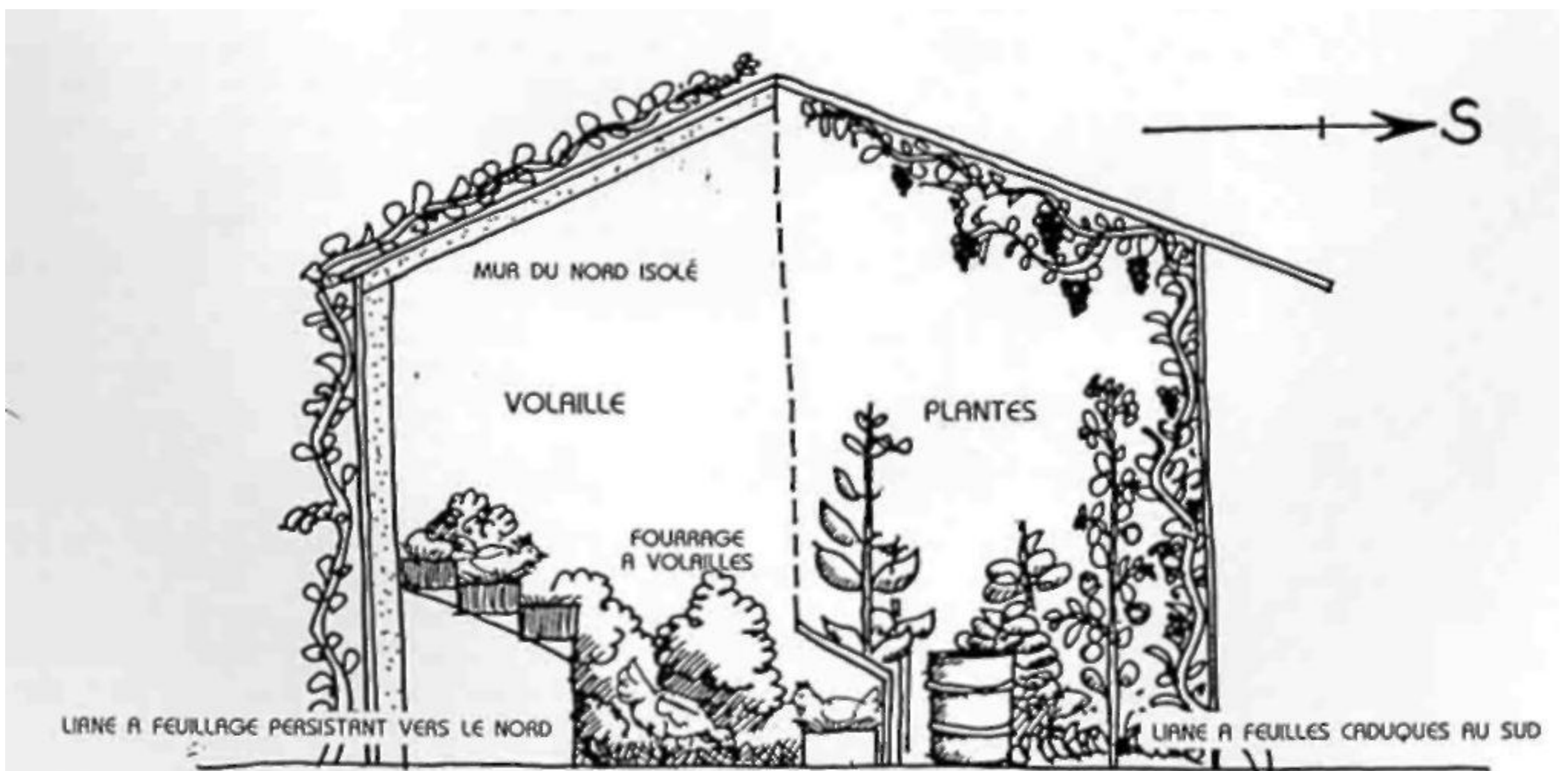
FIG. 8.3 : SERRE CHAUFFÉE PAR LES POULES.
