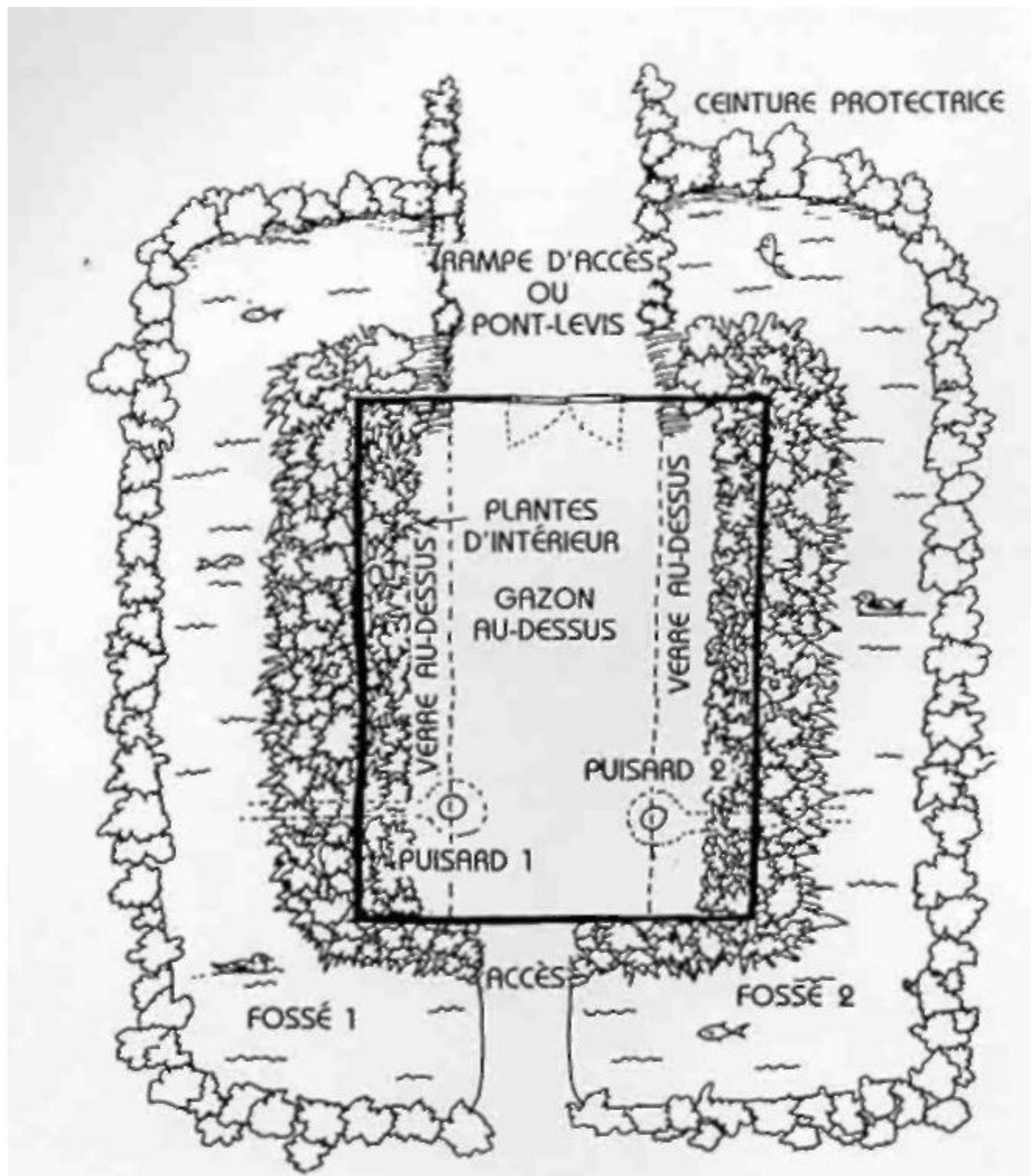
FIG. 6.7 : PLAN D'UNE MAISON DE TERRE CONÇUE POUR LA TOUNDRA OU DES PLAINES VENTÉES.
