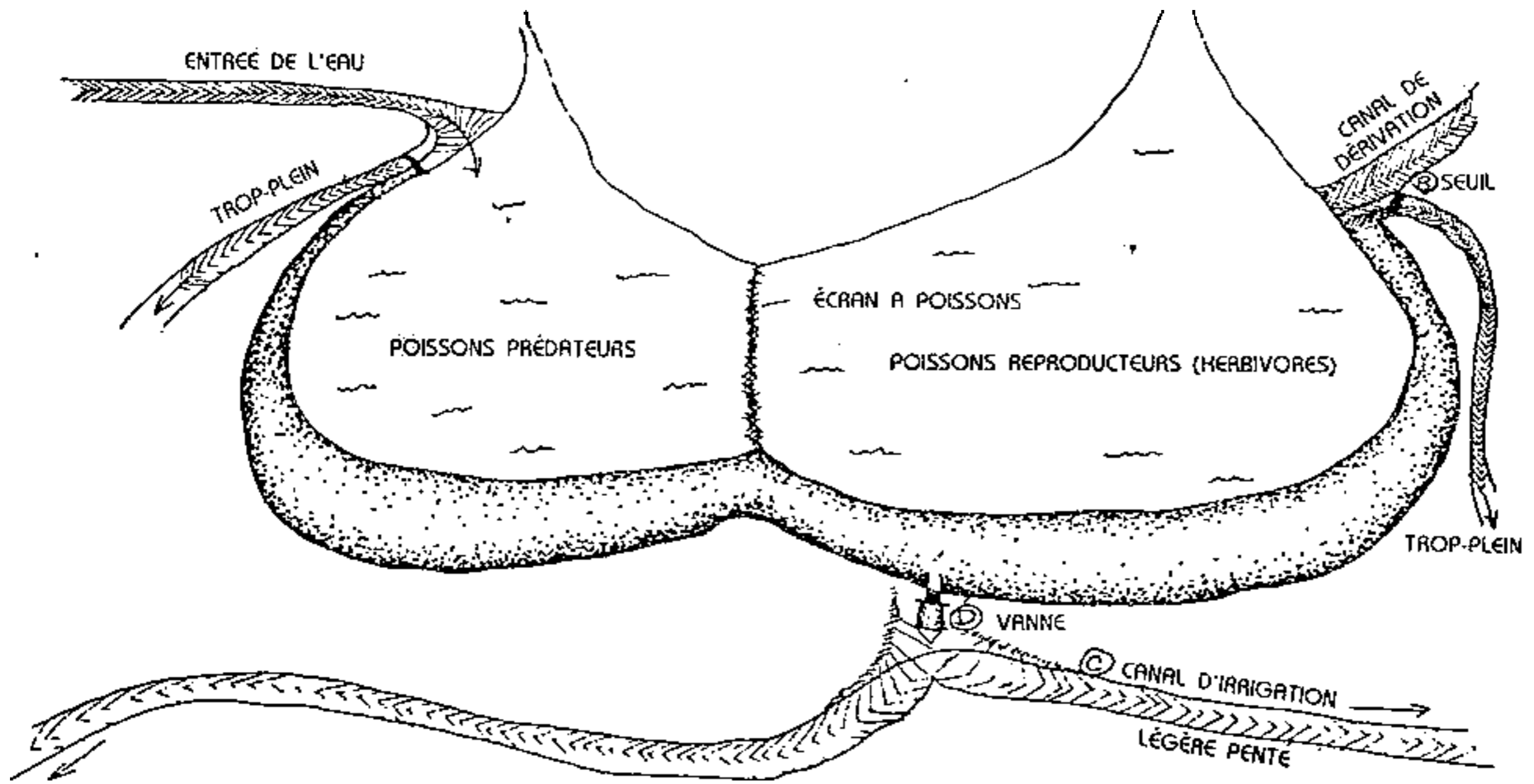
FIG. 7.12 : « DOUBLE » BARRAGE DANS UNE DÉPRESSION. LES DEUX PARTIES SONT CONNÉCTÉES PAR UN ÉCRAN A POISSONS. LES PRÉDATEURS (TRUITES) CONTRÔLENT LE NOMBRE DES HERBIVORES (PERCHES) AU MOYEN DE L'ÉCRAN A POISSONS (YANDOIT, VICTORIA).
