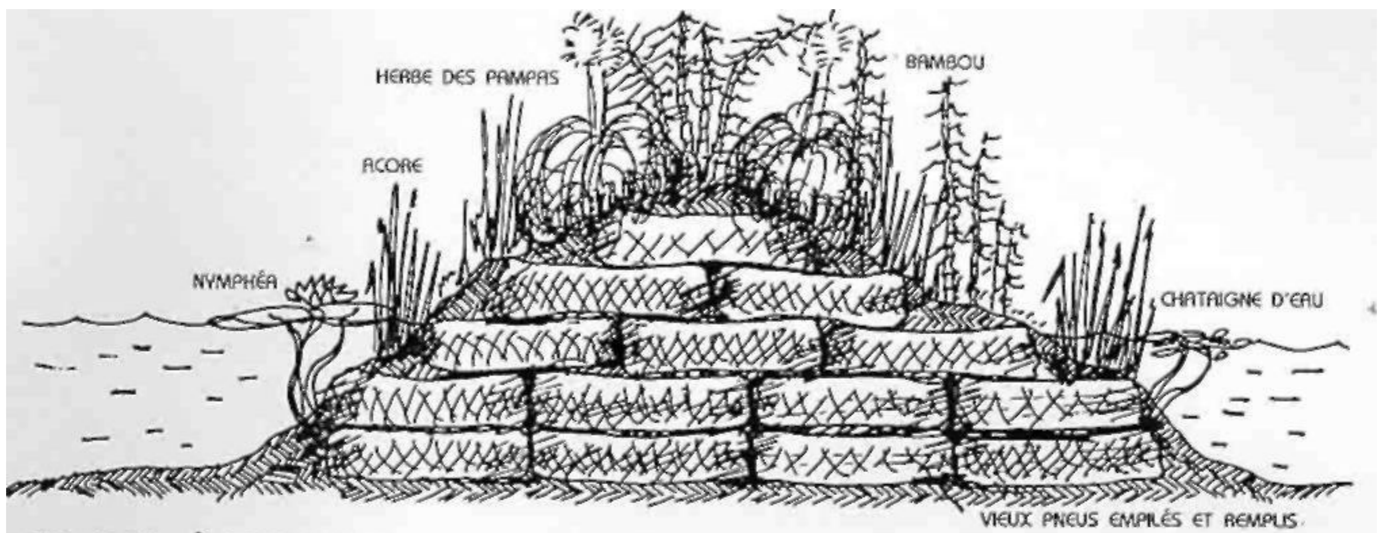
FIG. 7.20 : ÎLE DE PNEUS.
