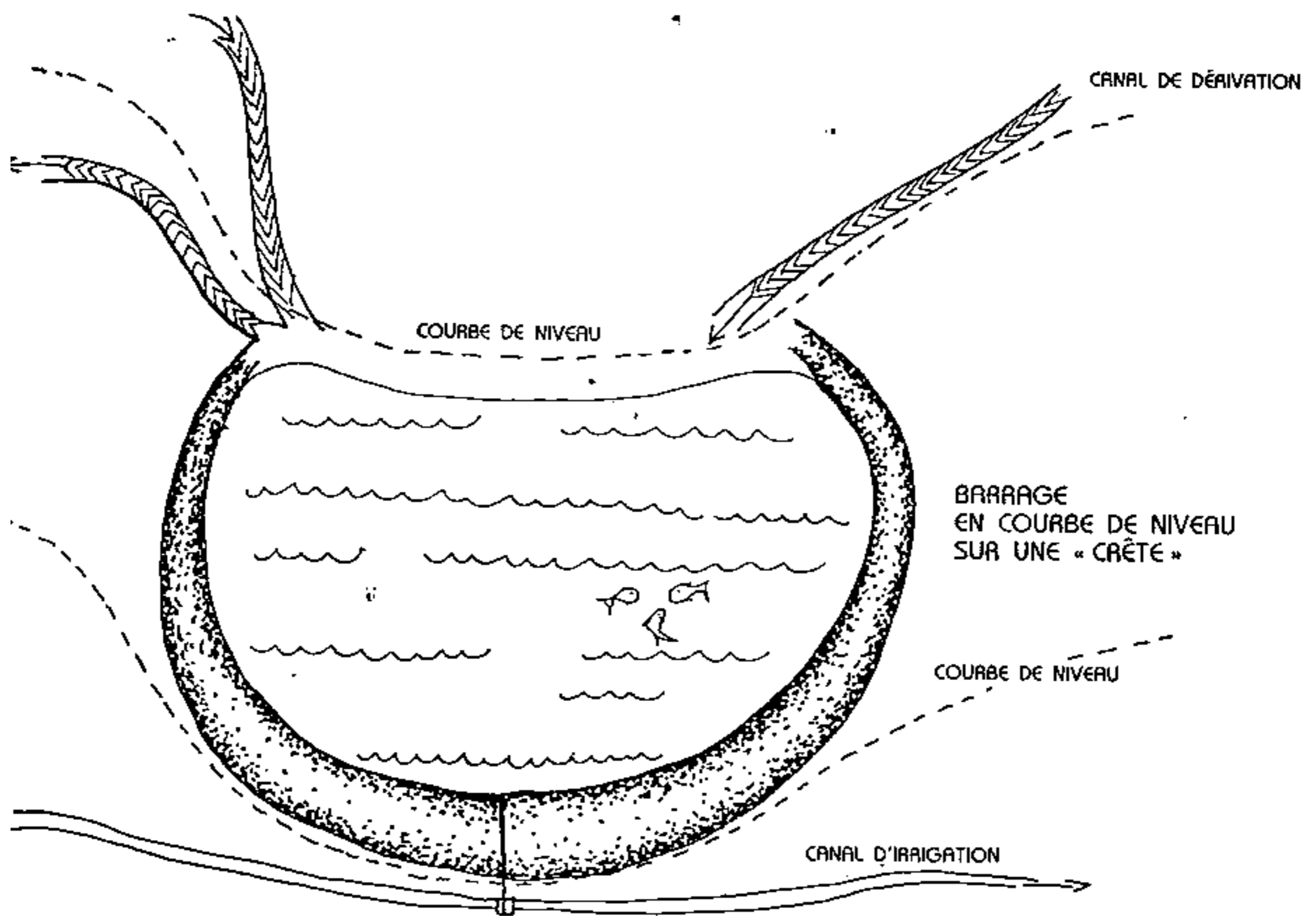
IG. 7.4 : BARRAGES EN COURBES DE NIVEAU.
